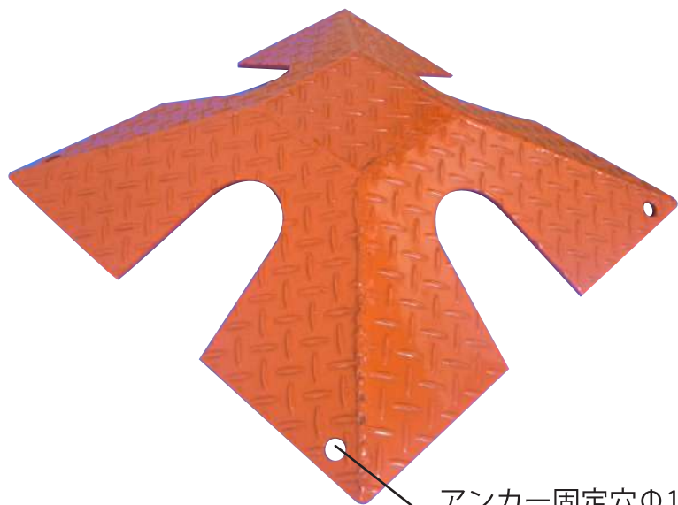
アンカー固定穴Φ14.5mm
